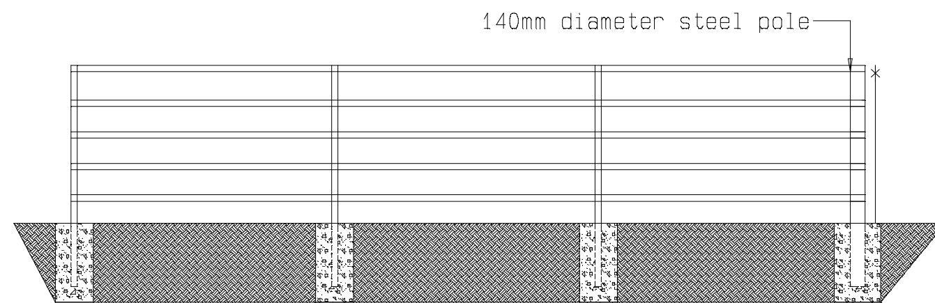
B- ELEVATION
